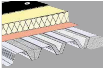
Sickenfüller
